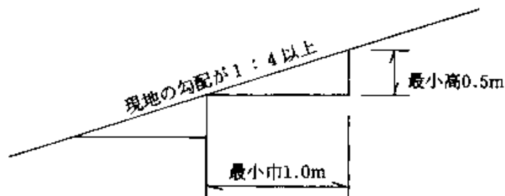
図2-1 盛土基礎地盤の段切
